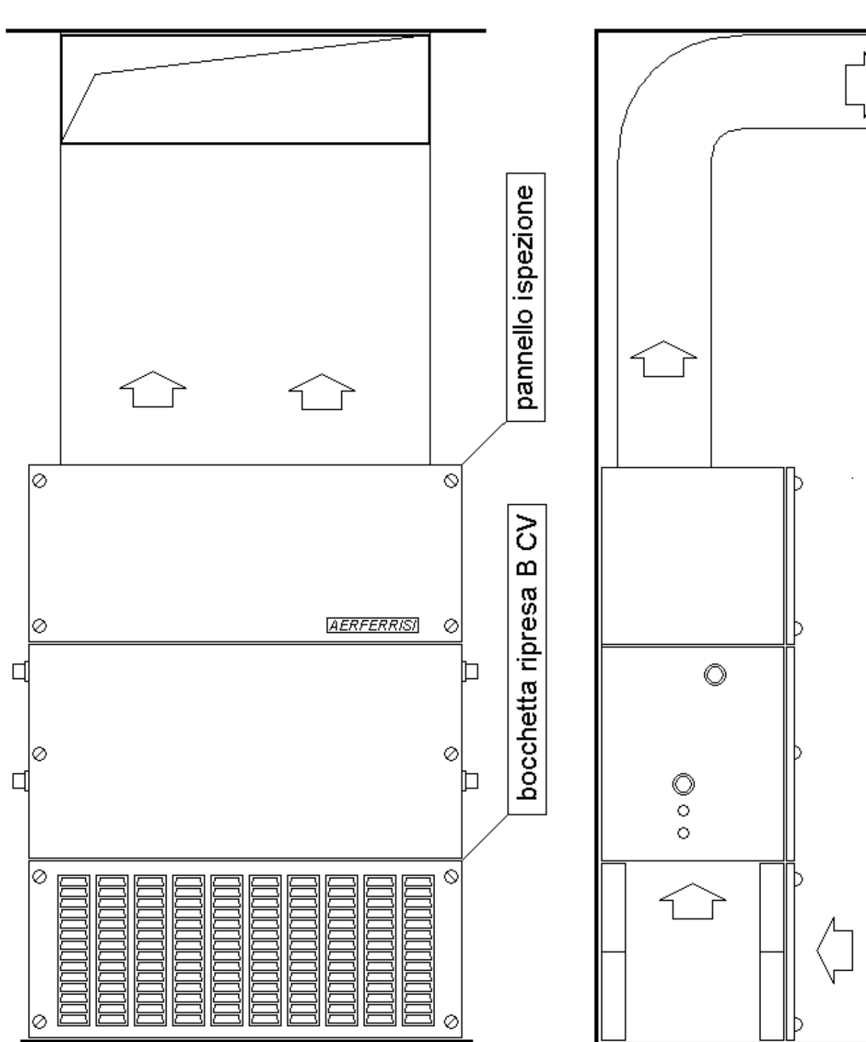
Montaggio con sola ripresa dall' ambiente
