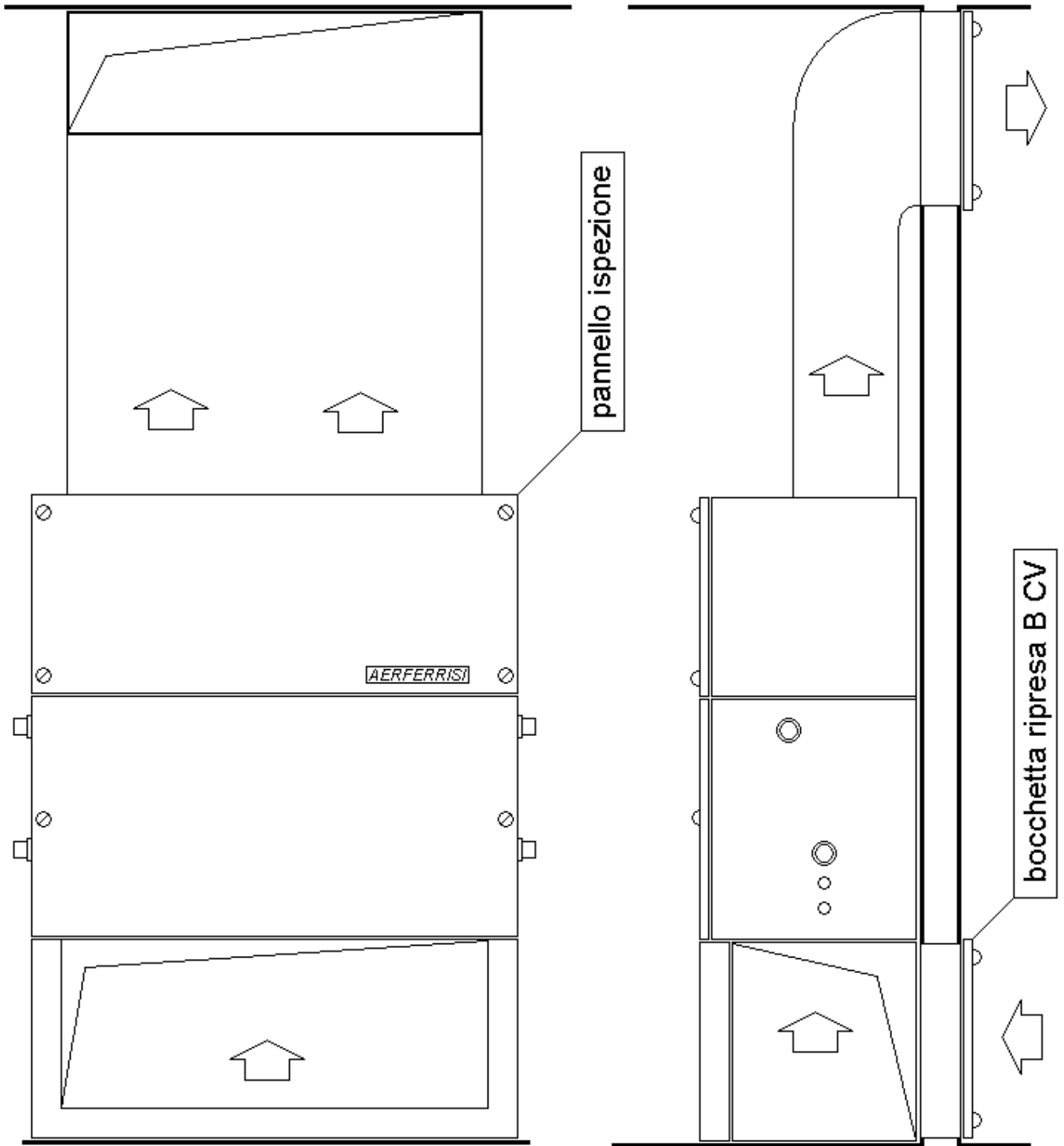
Montaggio a bocca libera in altro ambiente
