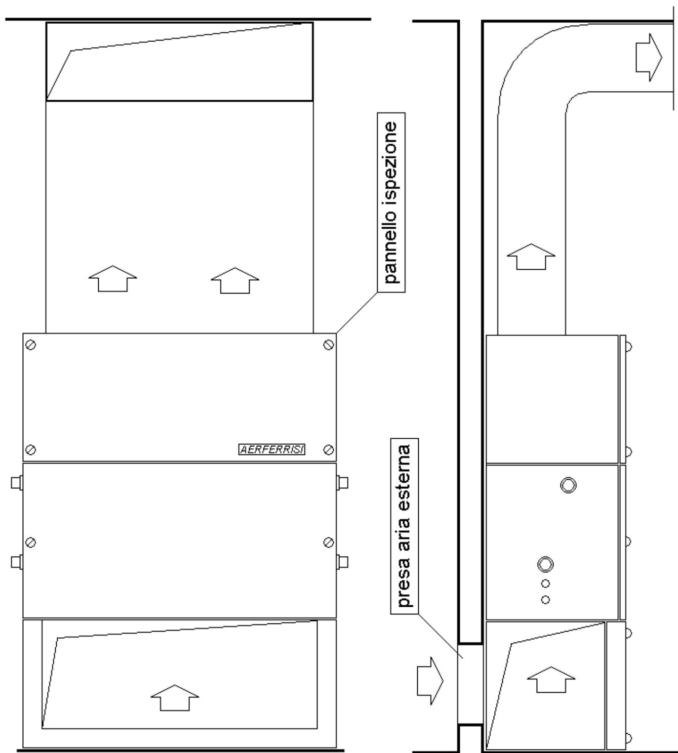
Montaggio con totale aria esterna
