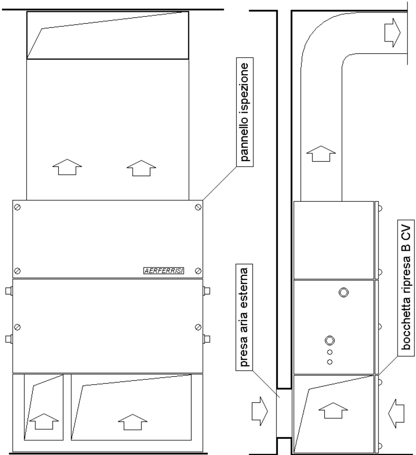
Montaggio con parziale aria esterna diretta
